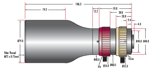
0.25X & 0.18X Telecentric Lenses
