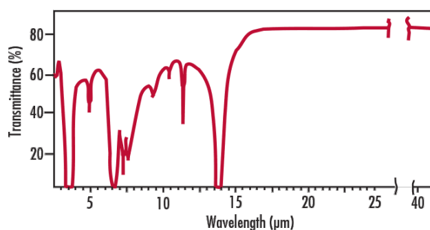
IR Windows in the IR Spectrum
