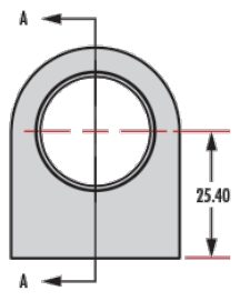
L-Slot Type (#36-410 & #36-416)
