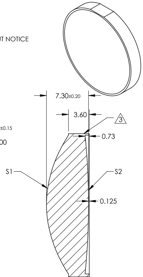
SECTION A-A
