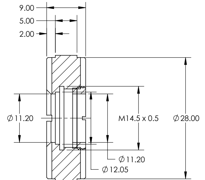
SECTION A-A
