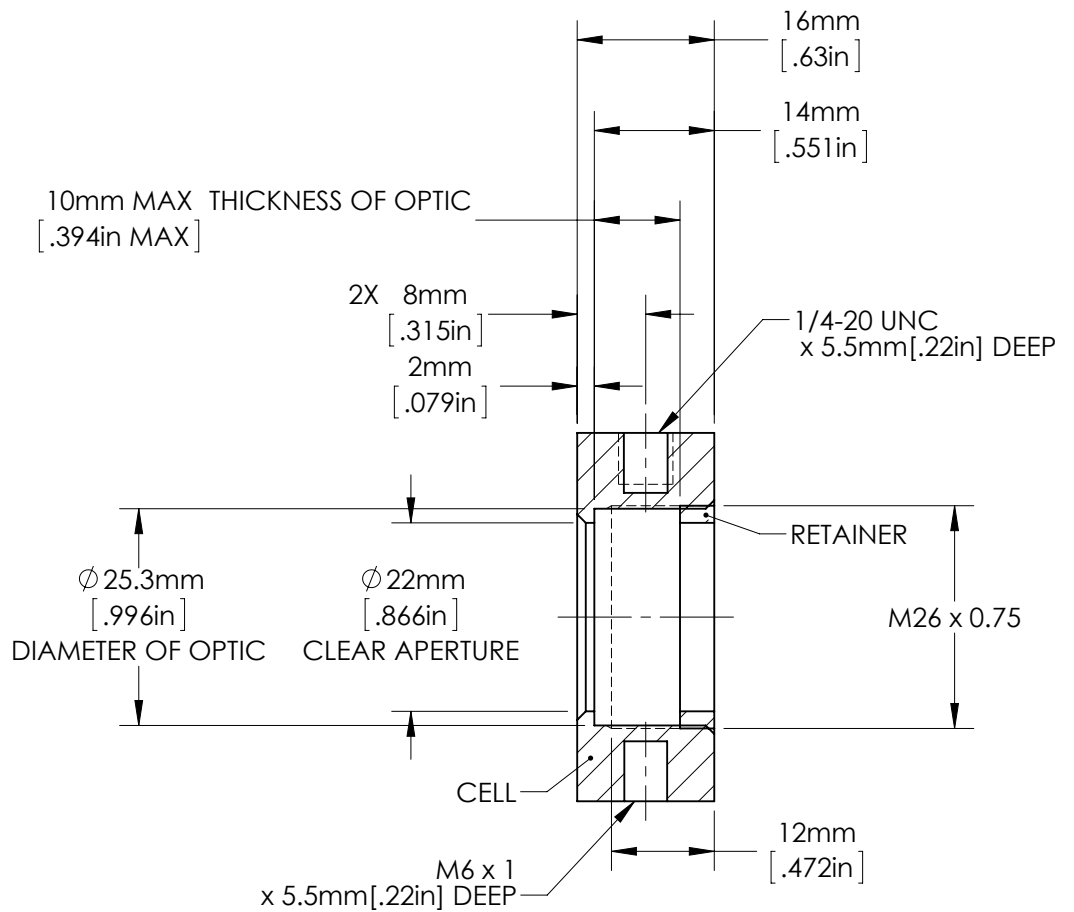
SECTION A-A
